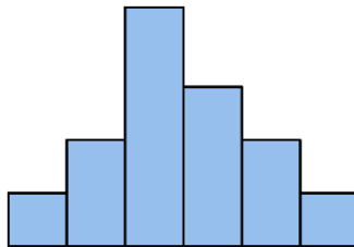
Figura 4. Función de distribución normal.
