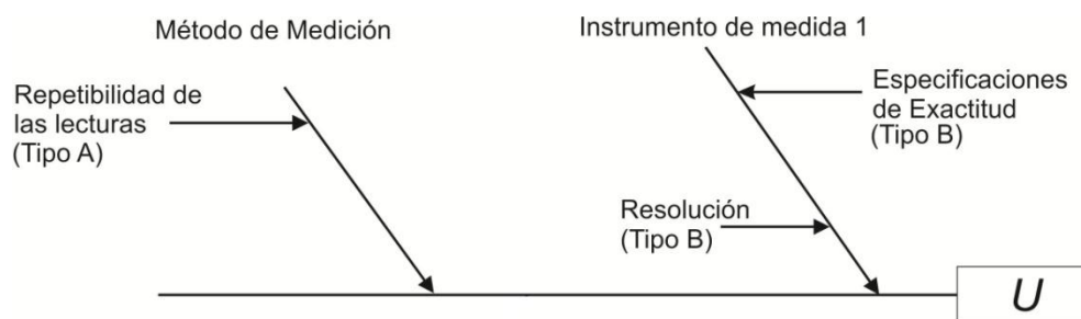
Figura 7. Fuentes de incertidumbre involucradas en el proceso de medición.
