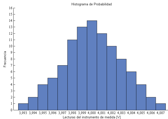
Figura 2. Histograma de Probabilidad.
