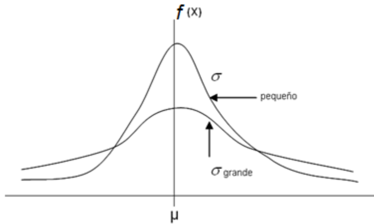
Figura 5. Curvas Gaussianas con diferentes \sigma .
