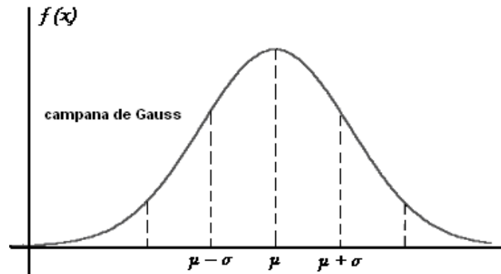
Figura 3. Distribución de probabilidades.
